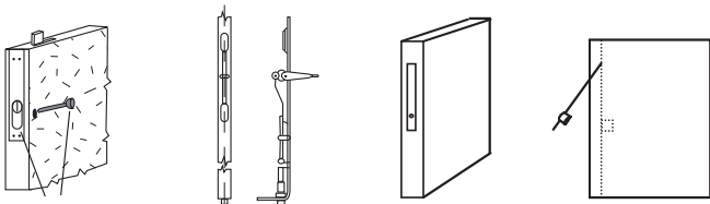
Gyűszűs tolzár rögzítése csavarral
