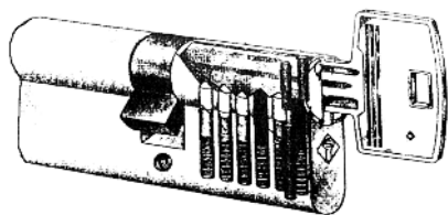
Biztonsági hengerezárbetét (6 csapos)
